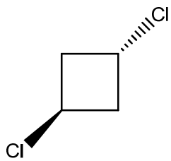
Trans- 1,3-diclorociclobutano
