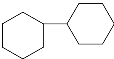
Cicloesilcicloesano
