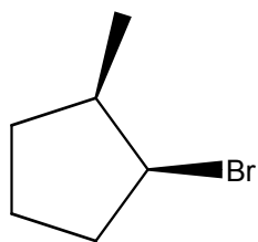
cis-2-bromo-1-metilciclopentano
